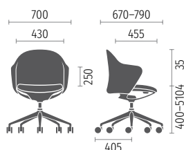
Base a 5 razze con rotelle
